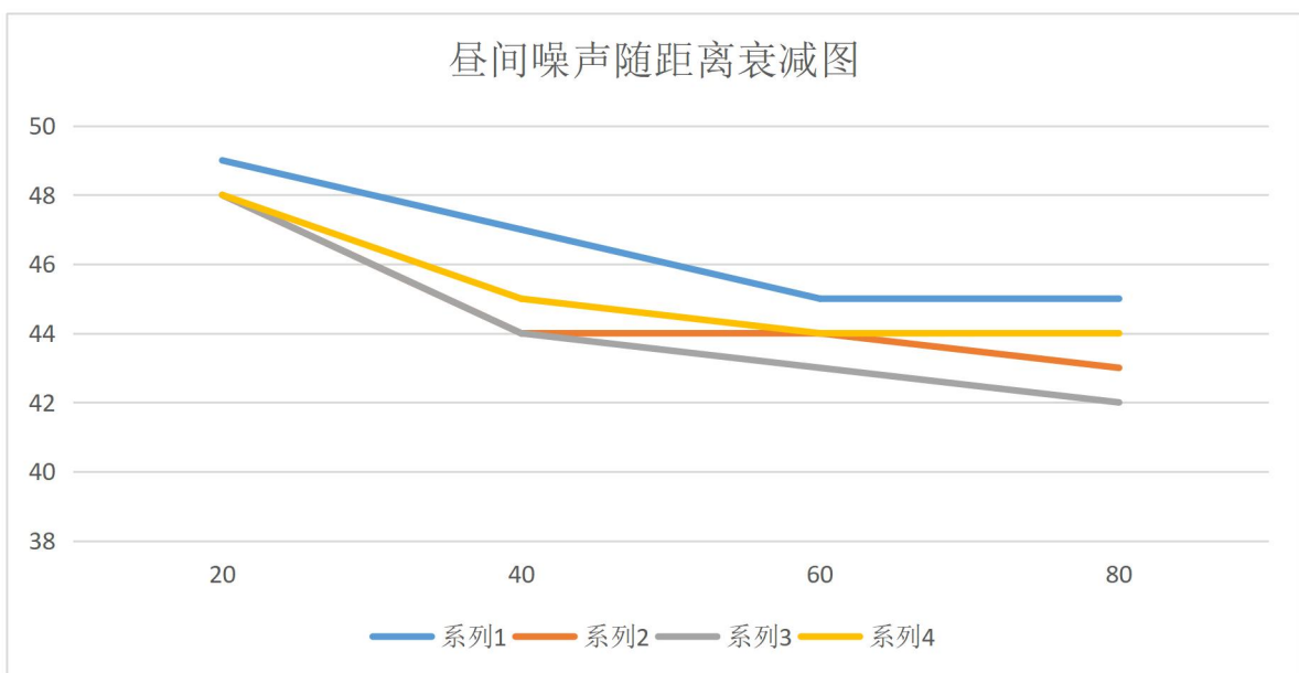
图 8-4 昼间噪声随距离衰减趋势图
