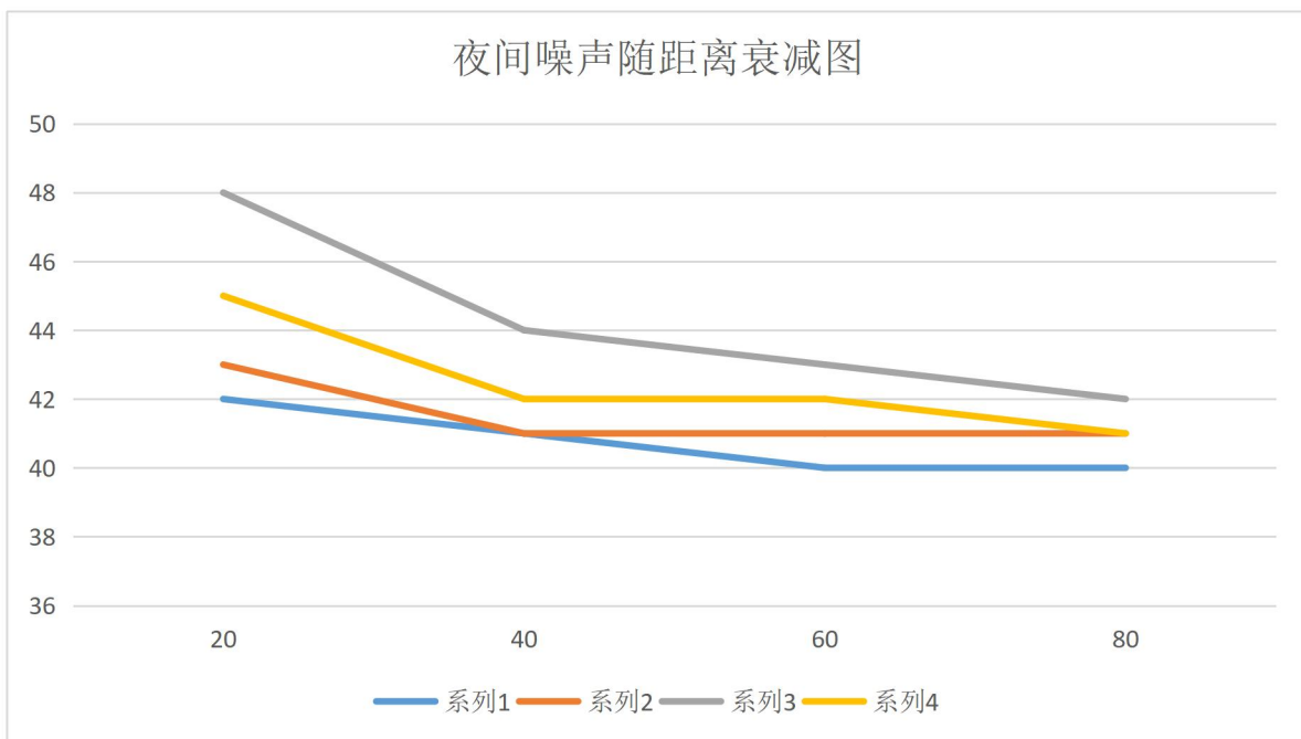
图 8-3 夜间噪声随距离衰减趋势图
