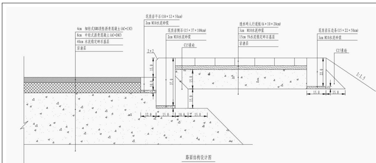
图 4-5 人行道道路结构图
