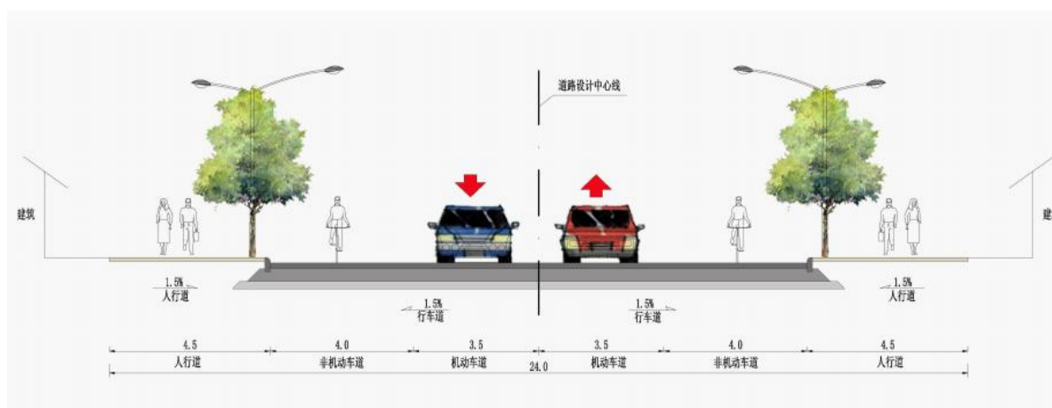
图 4-4 本项目道路横断面结构图
