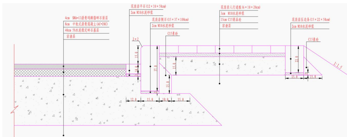
图 4-4 车行道路面结构图
