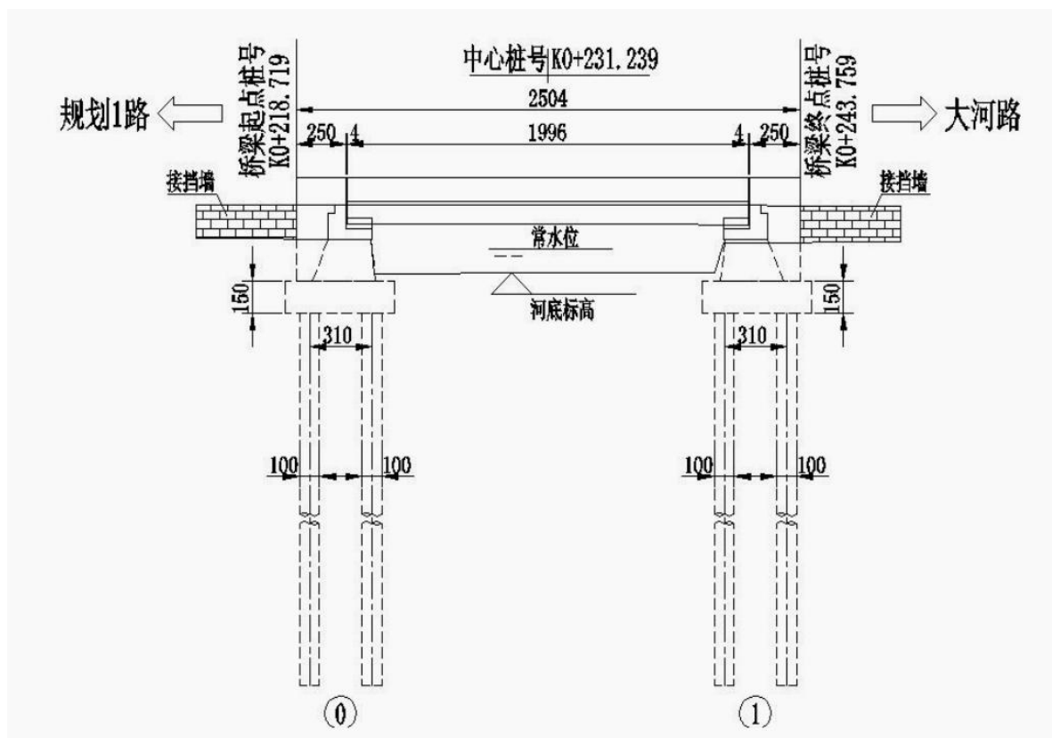
图 4-7 本项目桥梁结构图
